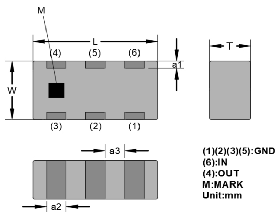
产品外形
